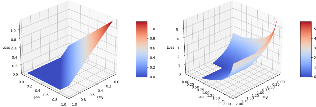
16. att. \mathcal{L}_{std} un \mathcal{L}_{exp} kļūdas funkciju salīdzinājums. Pozitīvie vienas klases pāru attālumi norādīti ar \|y_a - y_p\|_2^2 (pos), negatīvie dažādu klašu attālumi ar \|y_a - y_n\|_2^2 (neg).
