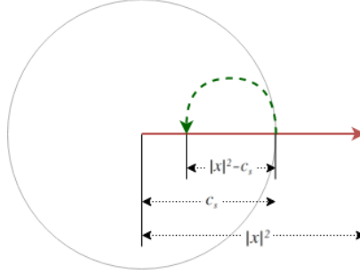
17. att. Unit-Bounce normalizācijas funkcijas ilustrācija latentajiem vektoriem eksponenciālajā trijotnes kļūdas funkcijā.
