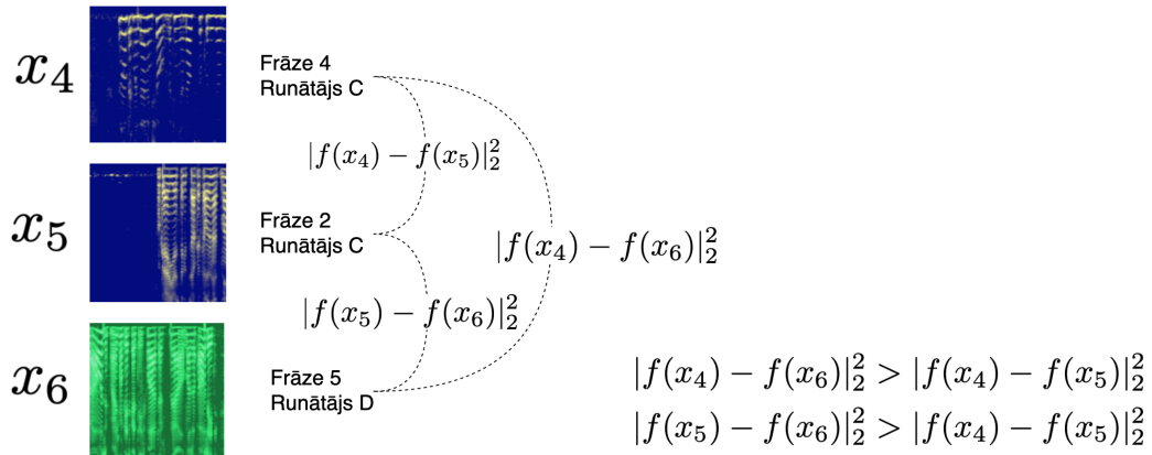
13. att. Atšķirība starp runātāja verifikācijas un runātāja reidentifikācijas uzdevumu (implementēts praktiskā lietojumā — komerciālā lietotnē "asya") Redentifikācijas uzdevums pieder pie nulles-šāviena apmācības, jo modelis f nav redzējis audio paraugus x_4, x_5, x_6 apmācības laikā.
